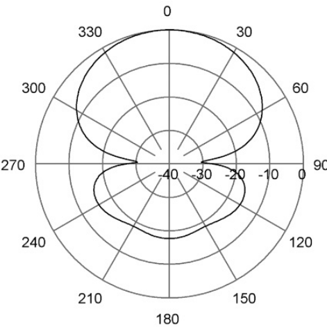
H-Plane | 400 MHz
