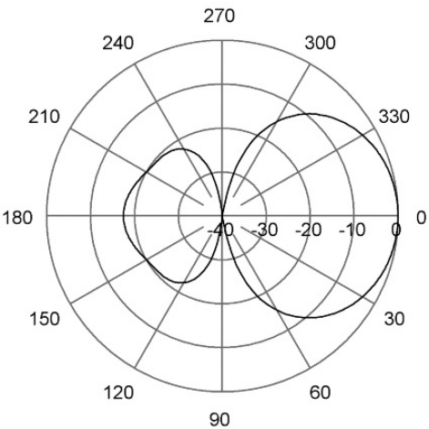
E-Plane | 400 MHz
