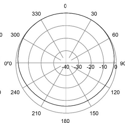
H-Plane | 158 MHz
