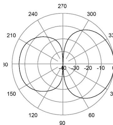
E-Plane | 158 MHz
