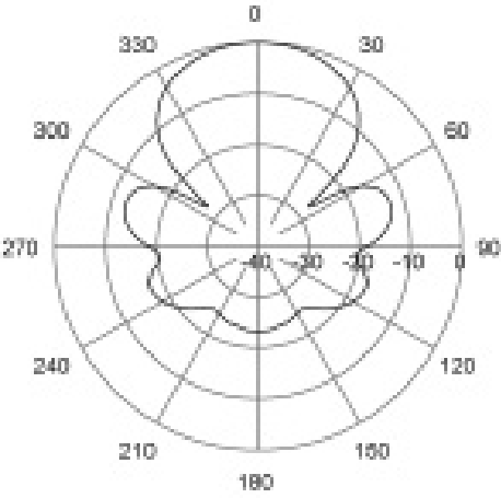
H-Plane | 405 MHz
