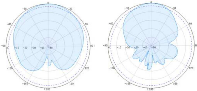
H-Pattern
