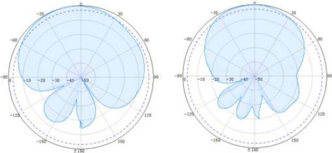
V-Pattern
