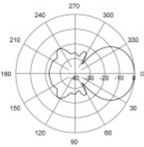
E-Plane | 445 MHz
