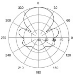
H-Plane | 445 MHz
