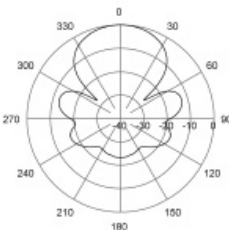
H-Plane | 155 MHz
