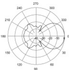
E-Plane | 155 MHz
