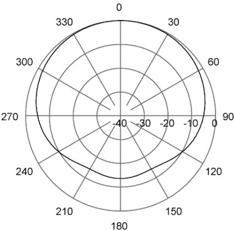
H-Plane | 445 MHz
