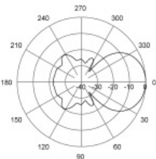
E-Plane | 165 MHz
