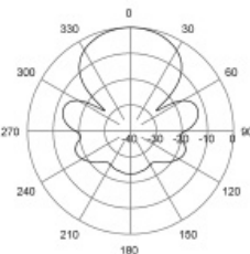
H-Plane | 165 MHz
