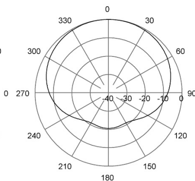
H-Plane | 152 MHz
