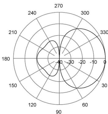
E-Plane | 152 MHz
