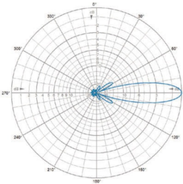
E-Plane | 425 MHz
