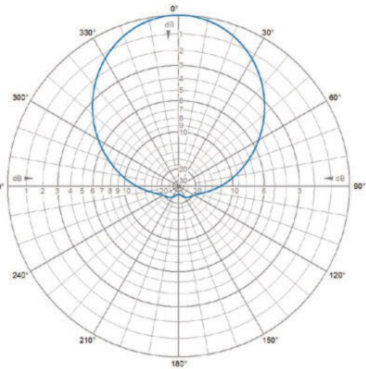
H-Plane | 425 MHz
