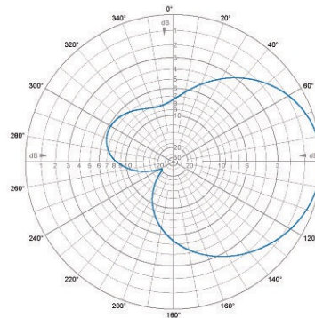
E-Plane | 425 MHz
