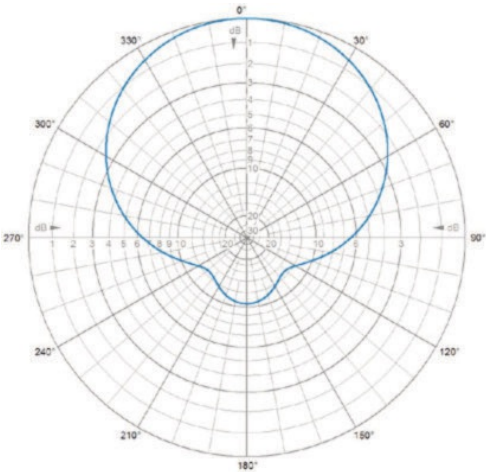
H-Plane | 405 MHz
