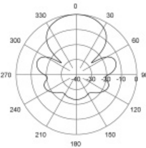
H-Plane | 395 MHz
